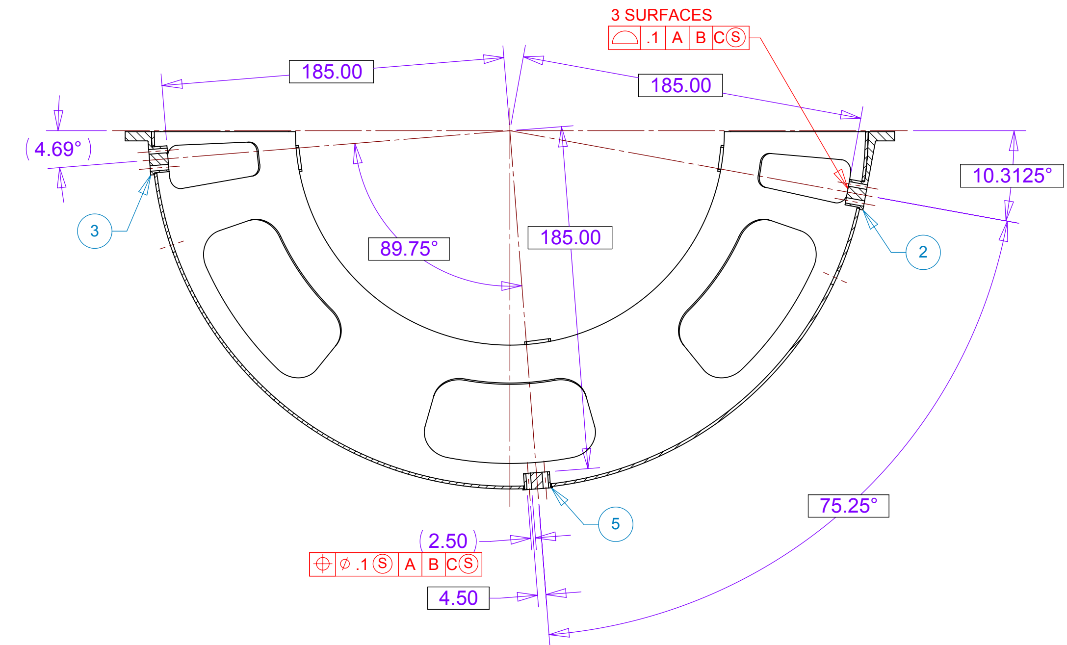
SECTION B-B SCALE 1 : 2
