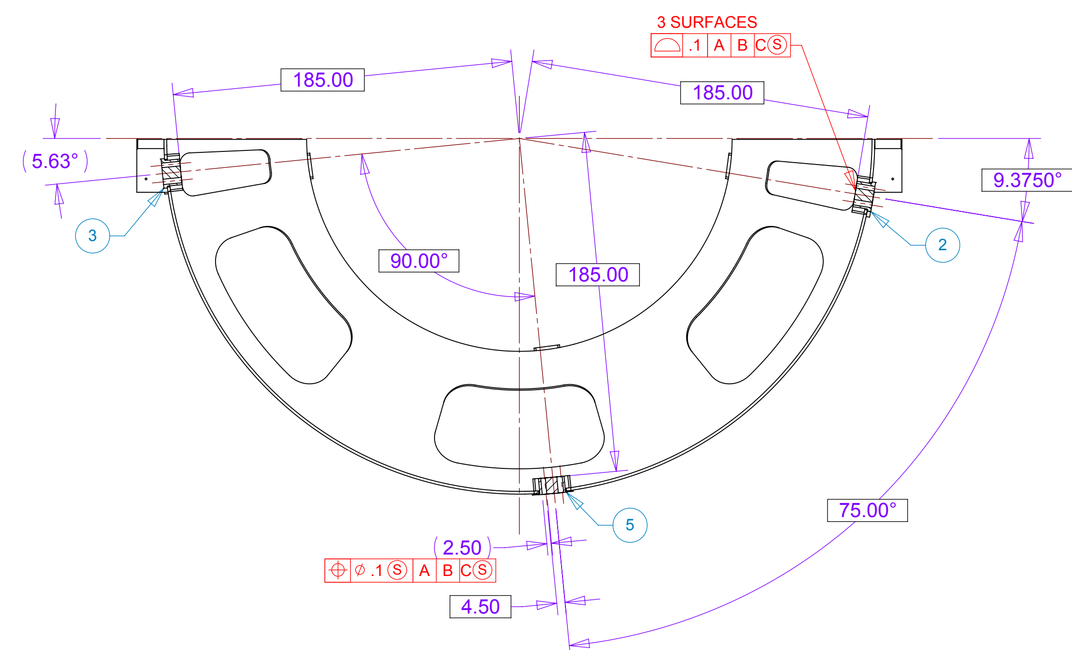
SECTION D-D SCALE 1 : 2
